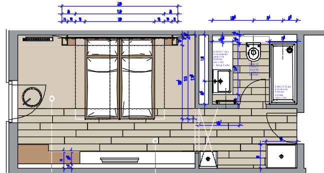
Grundriss Hotelzimmer / Flur
